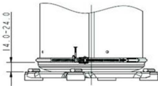
ZR84-144KC ZP90-137KC
